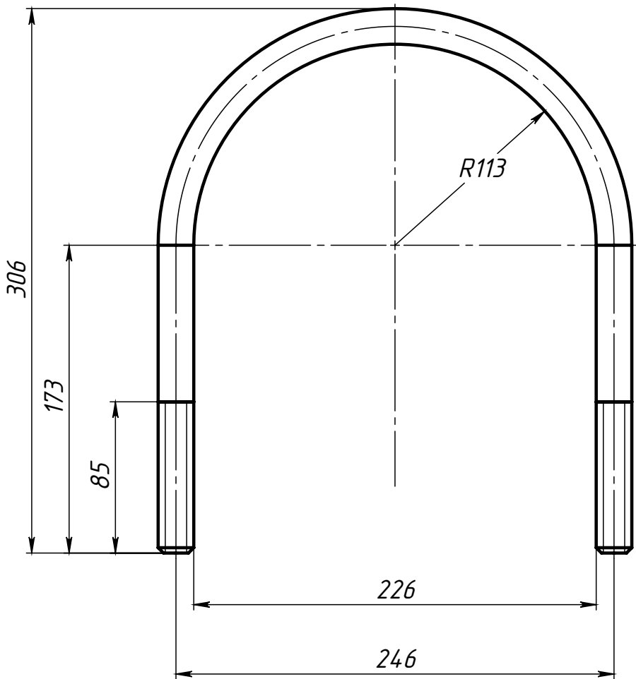
Поз.2 (Хомут)
