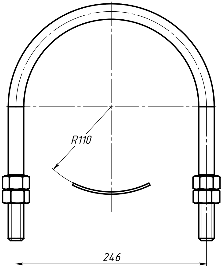
Поз.2 (Хомут)
